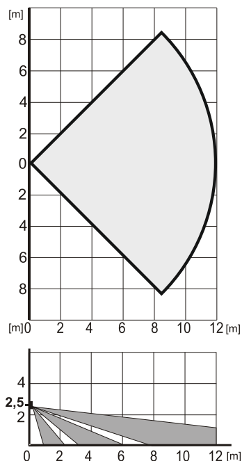
Rysunek 3. Charakterystyka detekcji czujki PIR
